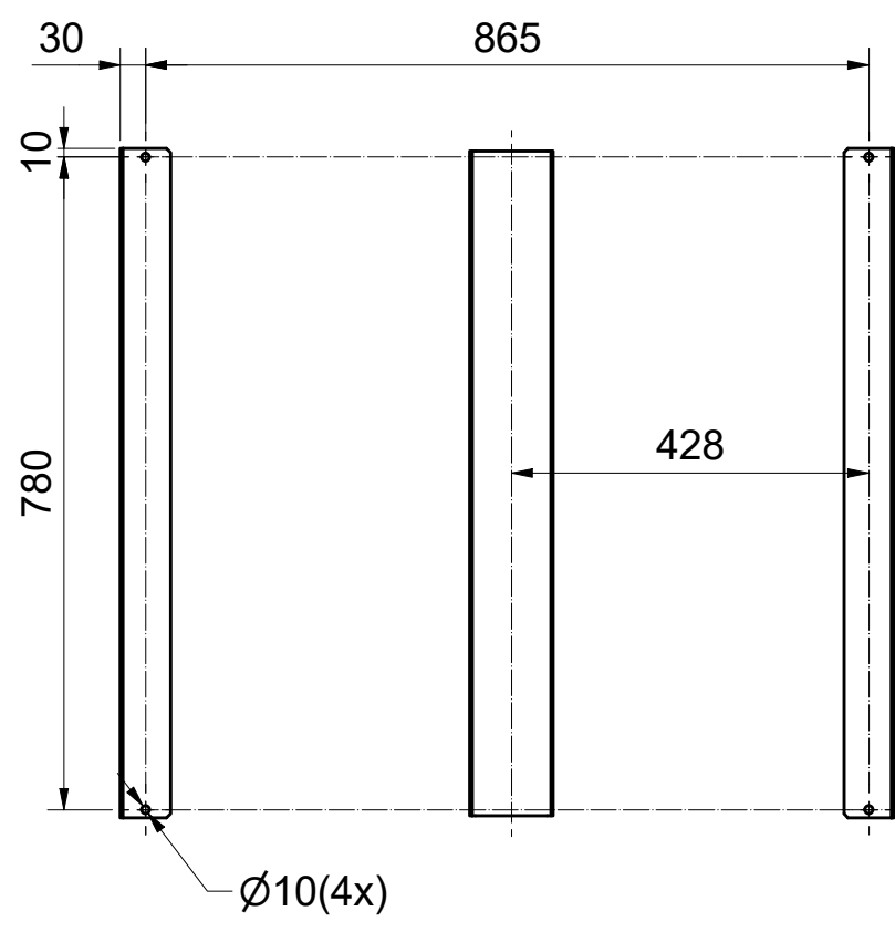
A-A ( 1 : 10 )
