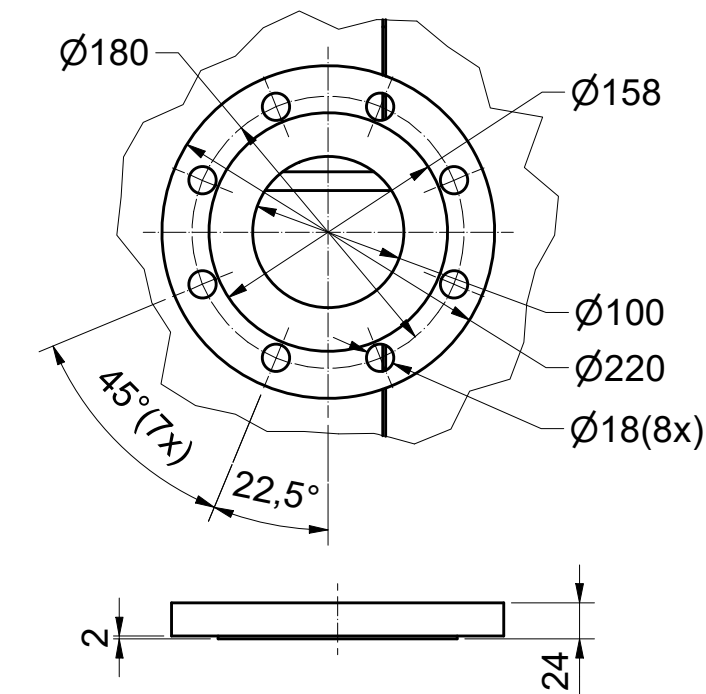
Detail of Inlet/outlet flange DN100 PN16A ( 1 : 5 ) (2x)
