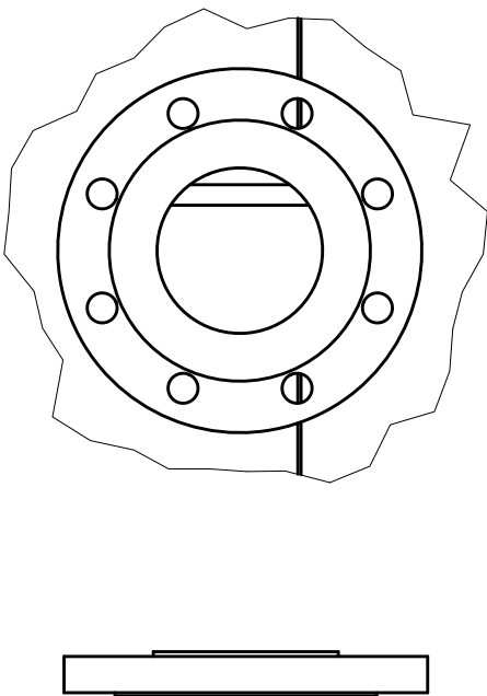
Detail of Inlet/outlet flange DN100 PN16A ( 1 : 5 ) (2x)
