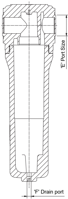
A-A (1 : 3)
