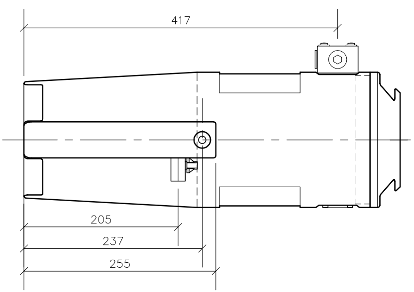
ELEVATION C-C
