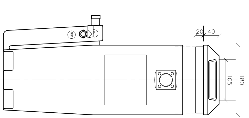
ELEVATION B-B
