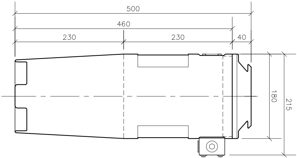
ELEVATION A-A
