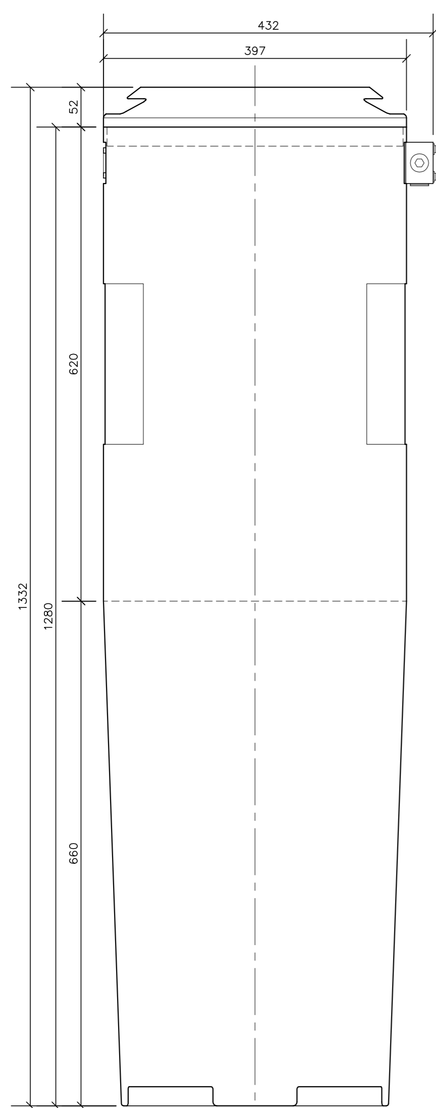
ELEVATION A-A
