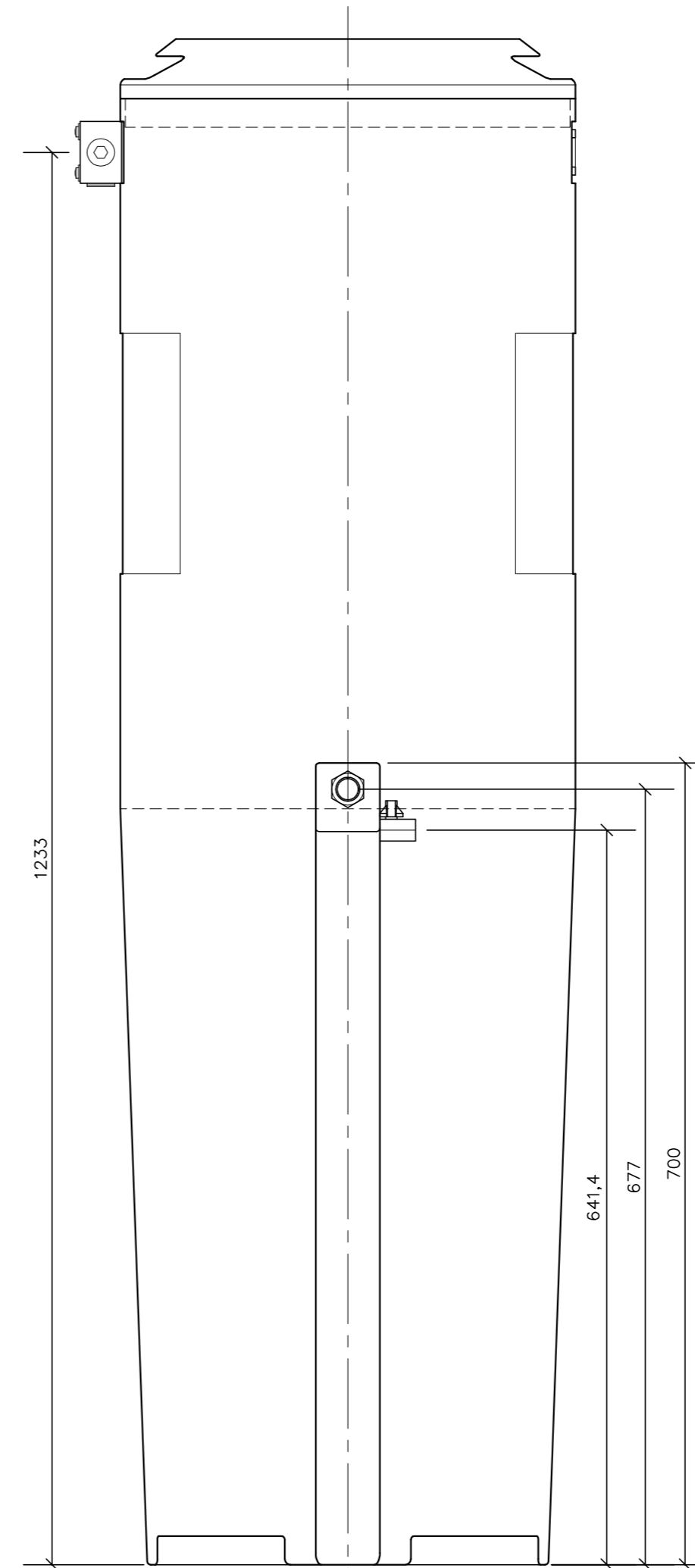
ELEVATION C-C
