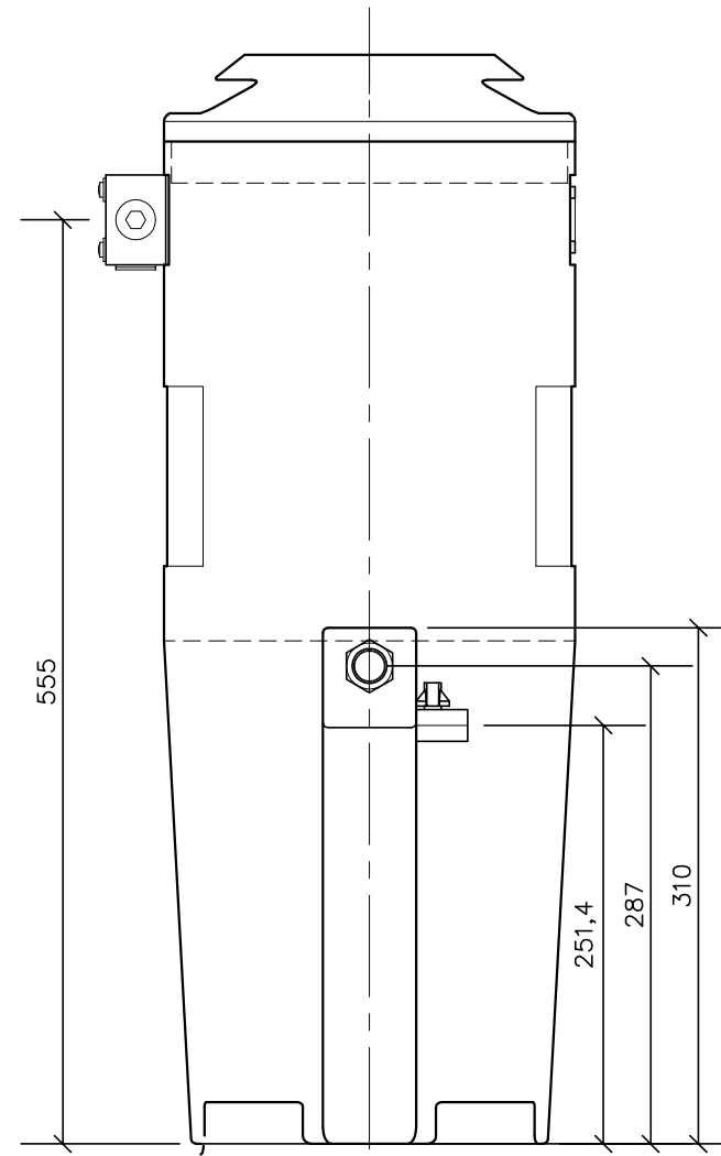
ELEVATION C-C
