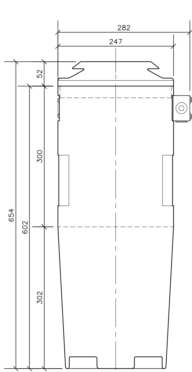
ELEVATION A-A
