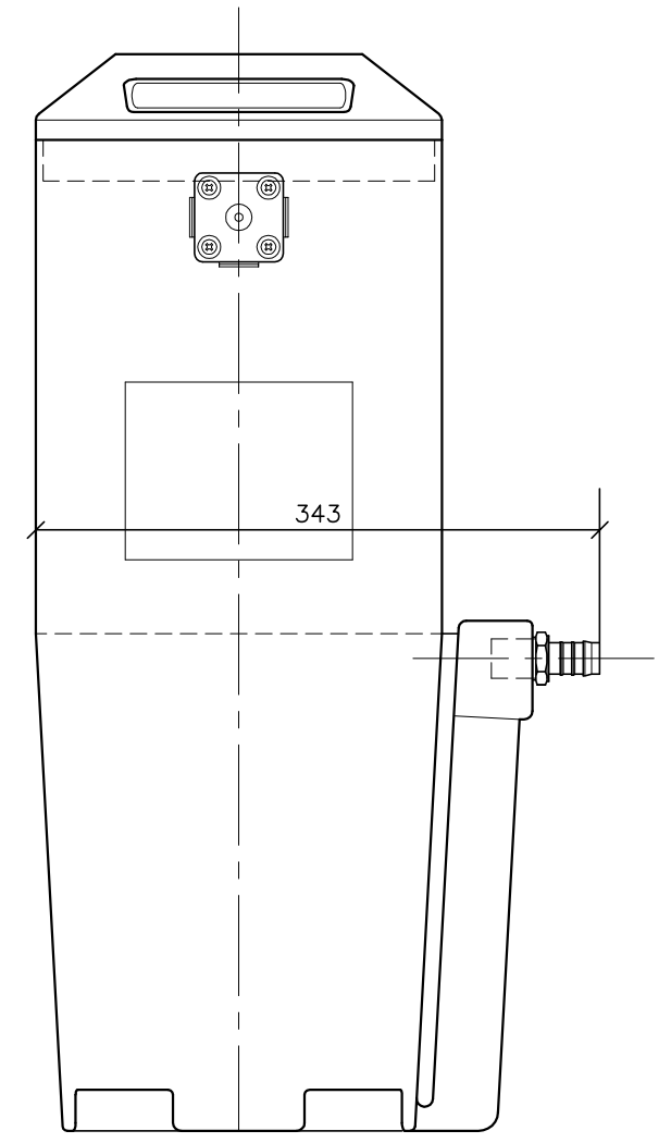
ELEVATION D-D
