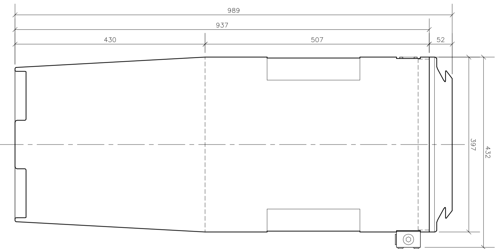
ELEVATION A-A
