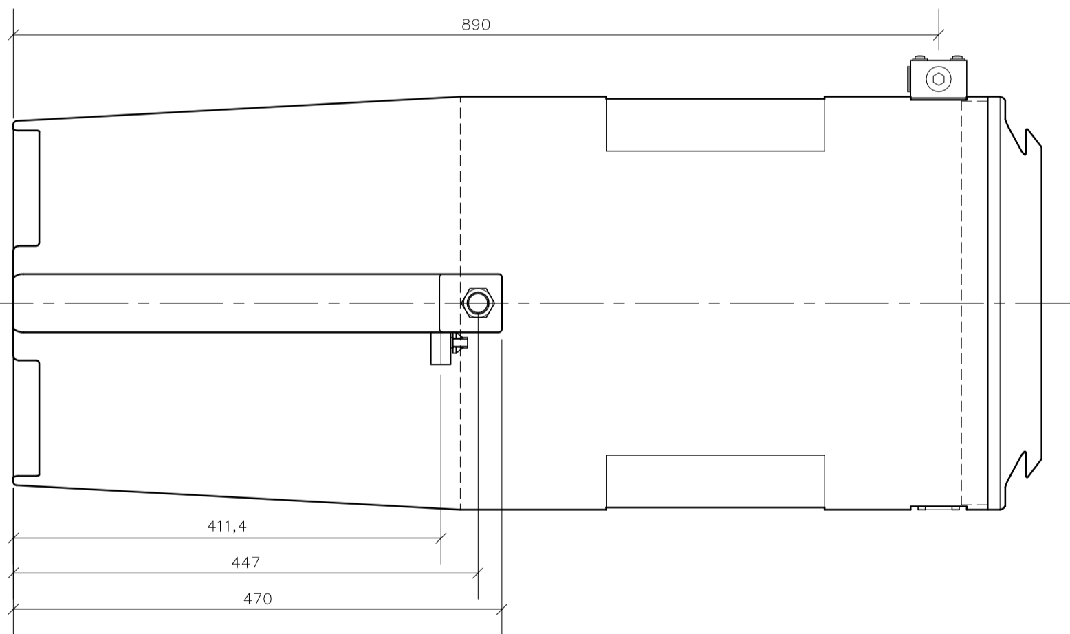
ELEVATION C-C
