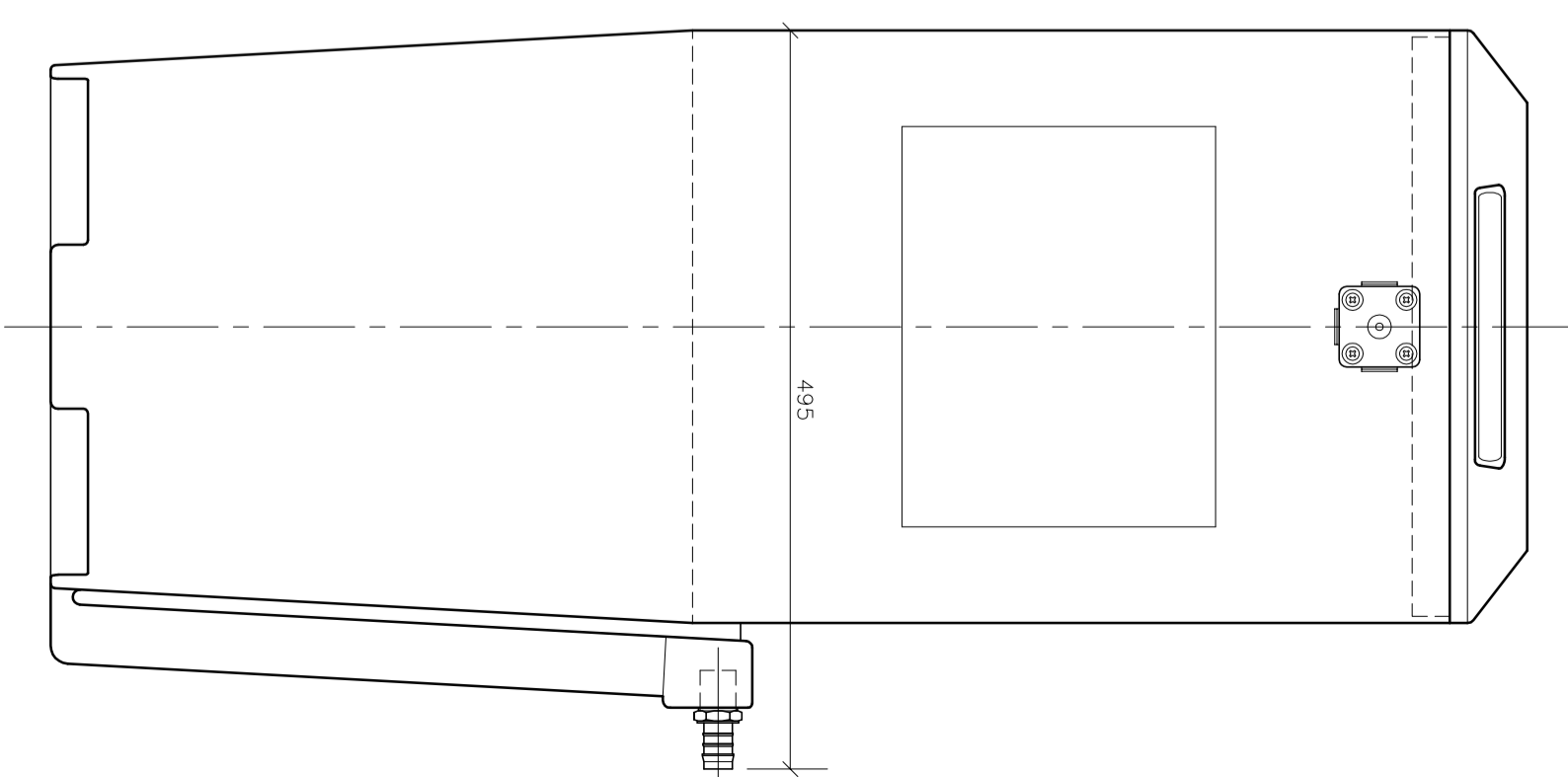
ELEVATION D-D
