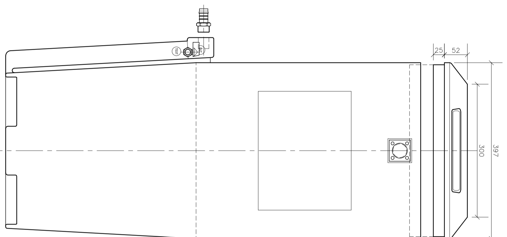
ELEVATION B-B
