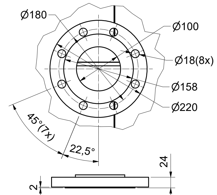
Detail of Inlet/outlet flange DN100 PN16A ( 1 : 5 ) (2x)
